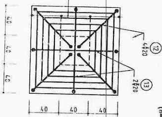
بش b-b SCALE 1:25
