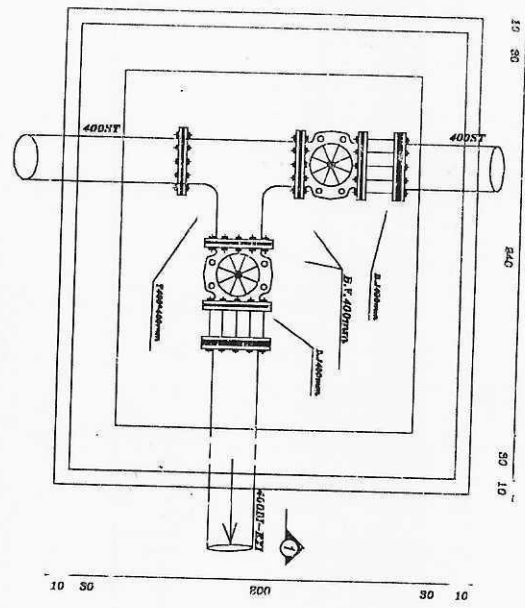
پلان حوضچه ورودی سیمان
